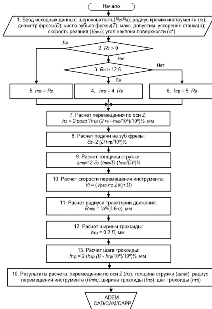
Рисунок 2.12 – Алгоритм комплексного решения проектных задач при автоматизированном проектировании высокоскоростной фрезерной обработки на станках с ЧПУ
